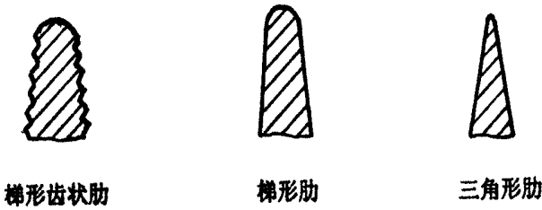
图 2 肋片截面形状
